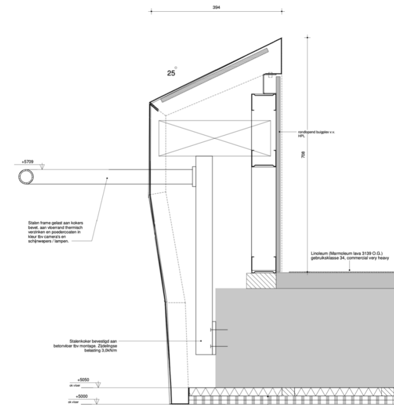
Figuur 1 dwarsdoorsnede balustrade t.p.v. de vloerrand van het theaterbalkon
