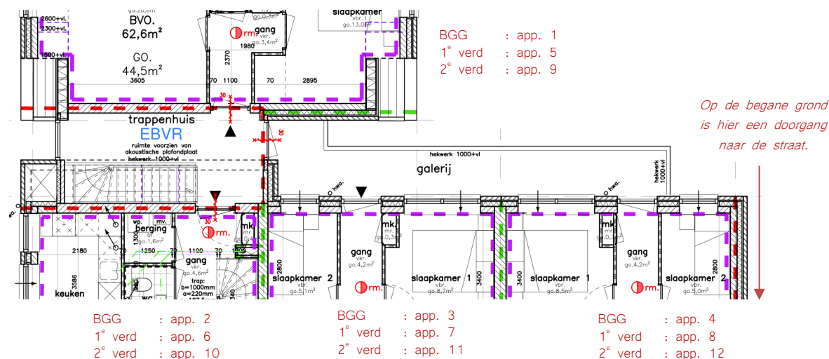
Figuur 1 Ontsluitingsprincipe appartementen. De vluchtroute van het meest rechter appartement voert altijd langs de naastliggende woning om het portiektrappenhuis te kunnen bereiken. De ontsluiting van de appartementen op de begane grond zijn recht onder de hier getekende ontsluitingen gepositioneerd, met uitzondering van het enkele appartement dat aan de bovenzijde van figuur 1 is weergegeven. Op de begane grond heeft die zijn ontsluiting verder naar rechts, buiten het portiektrappenhuis.
